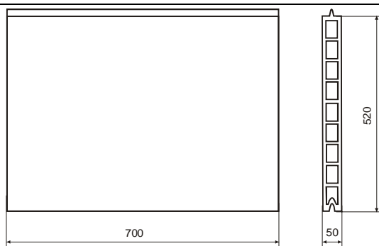
Croquis de la pieza Cotas en mm
